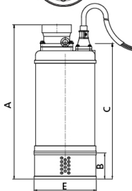
100(150) EUB-5.200~300
